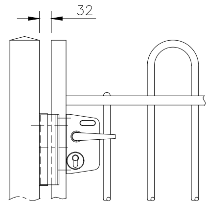
OPTIONAL KEY LOCK (SCALE 1:10)
